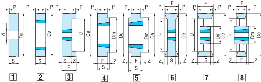
POULIES PPL à moyeu amovible PPL MA x D x nb gorges G
